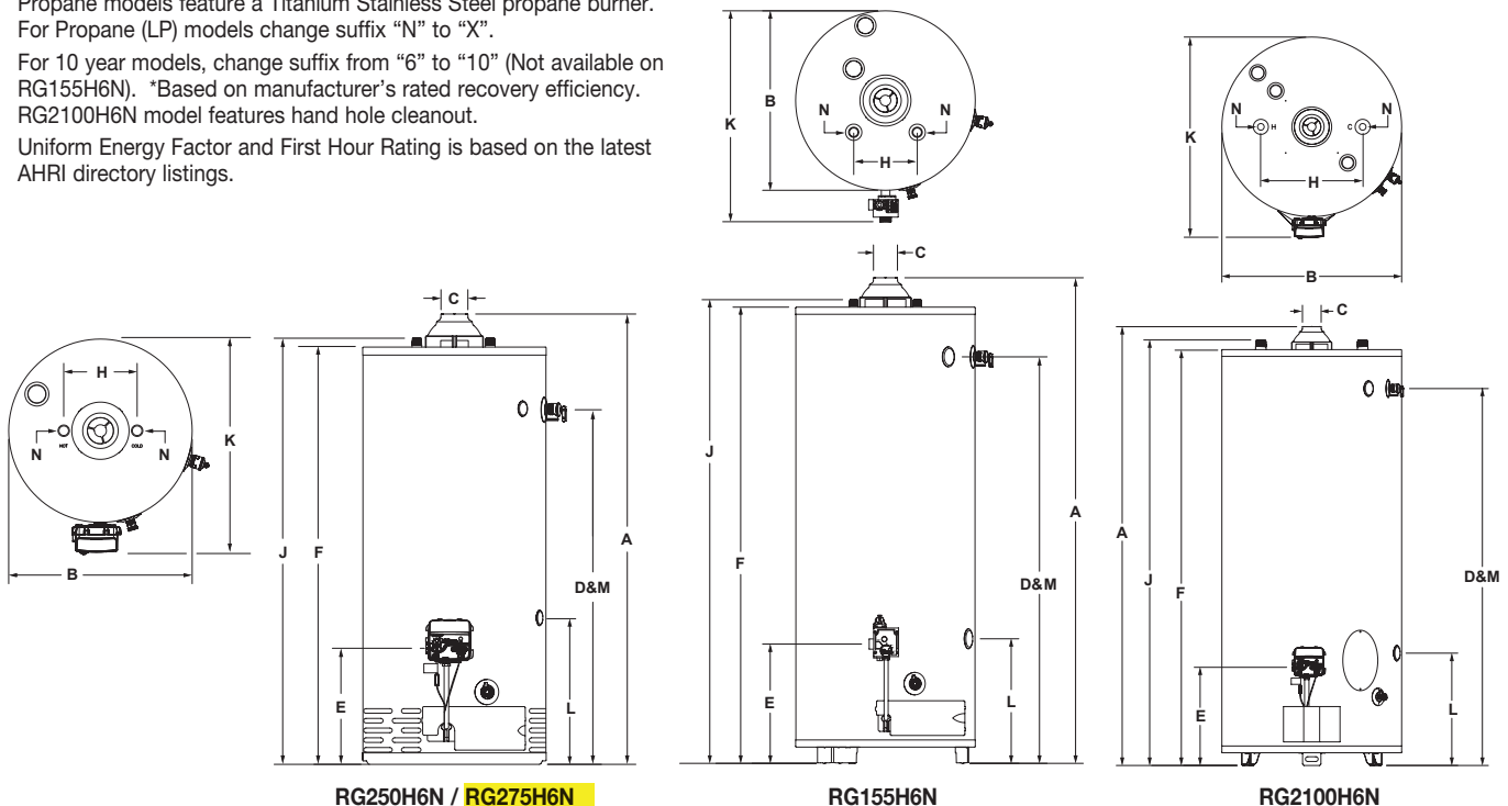
RG250H6N / RG275H6N
